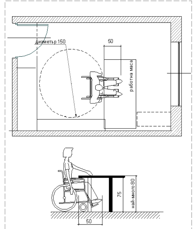
Фиг. 36. Оразмеряване на достъпно работно място
